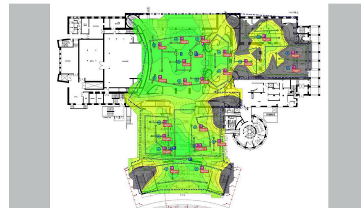
Abb. 3: IST-Zustand des WLANs im Erdgeschoss bei 2,4 GHz. Grüne Bereiche haben dabei über -42dBm, graue Bereiche sind zu optimieren.
