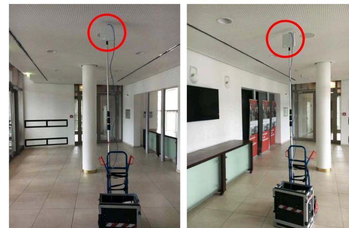
Abb. 7: Bei der Vorort-Messung wird eine mobile Einheit eingesetzt, um in allen Räumlichkeiten die WLAN-Parameter aufzunehmen.
