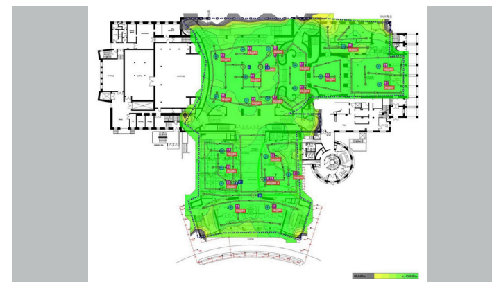
Abb. 4: SOLL-Zustand (Plan) im Erdgeschoss bei 2,4 GHz. Alle Bereiche sollen ausreichend mit WLAN versorgt werden.
